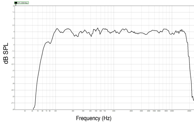
CPL1296zR 未经处理频率响应
