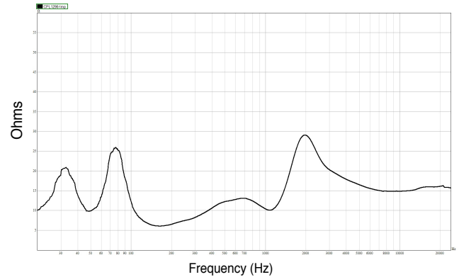
CPL1296zR 阻抗 VS. 频率
